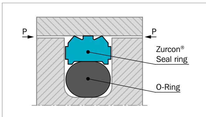
Figure 144: Zurcon® Wynseal
