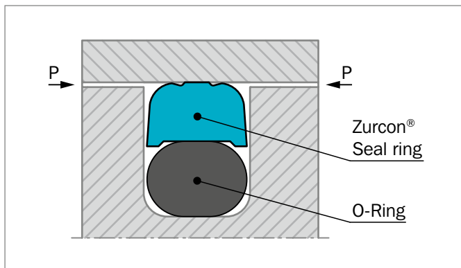
Figure 114: Zurcon® Glyd Ring® D
